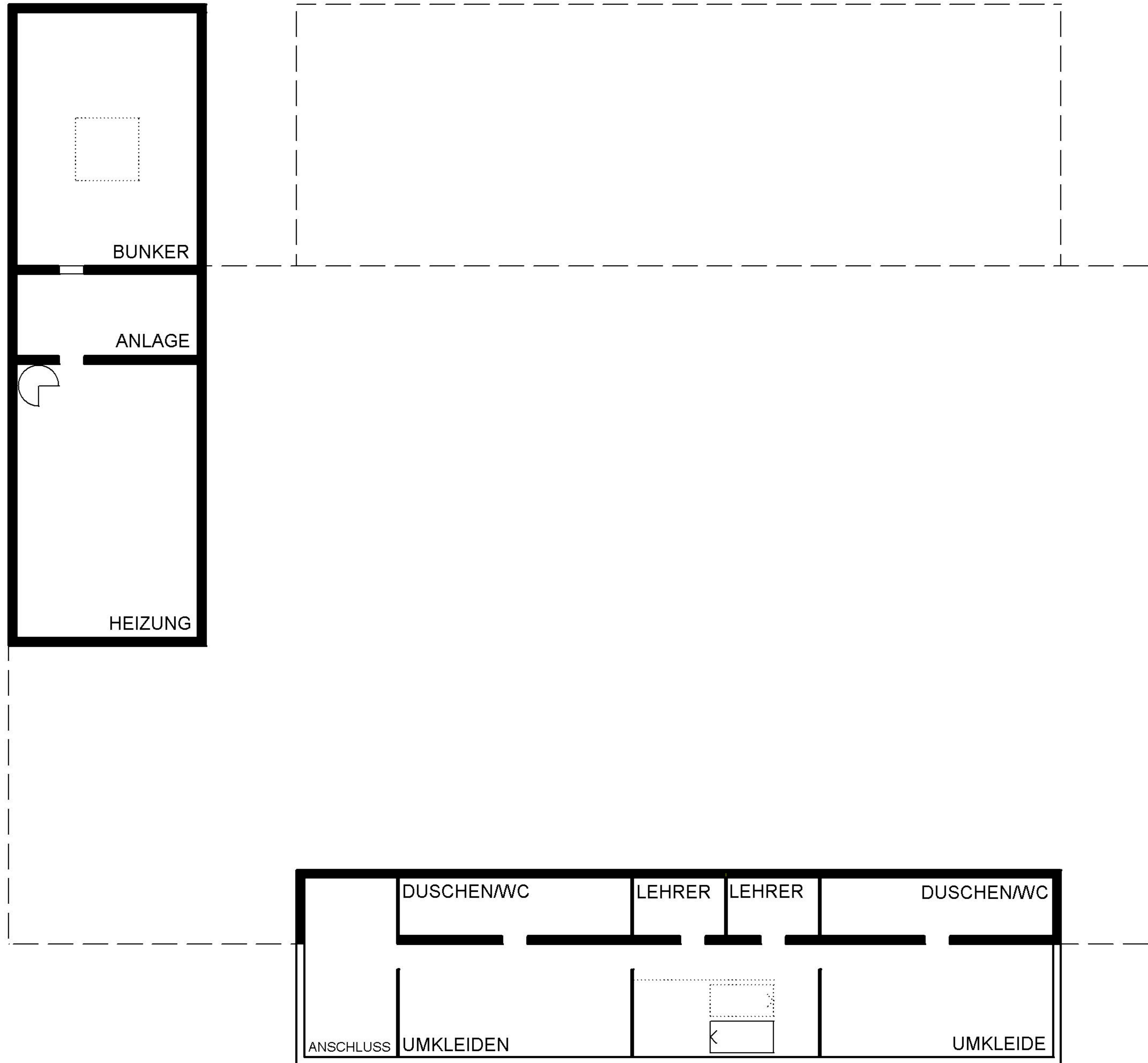
GRUNDRISS UG
