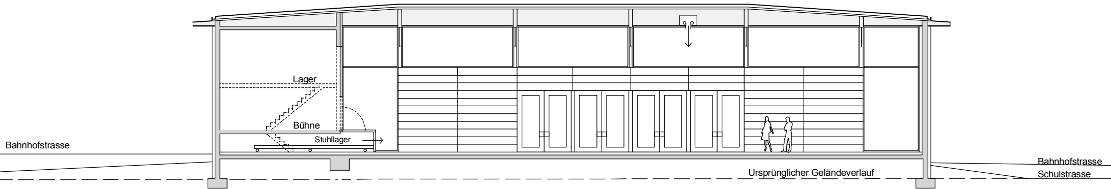
Schnitt B-B
