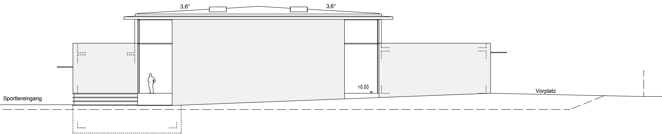
Ansicht Ost
